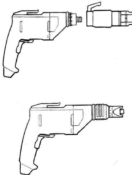
Pav. 15: Daugiasluoksnių statybinių plokščių savisriegių suktuvas
