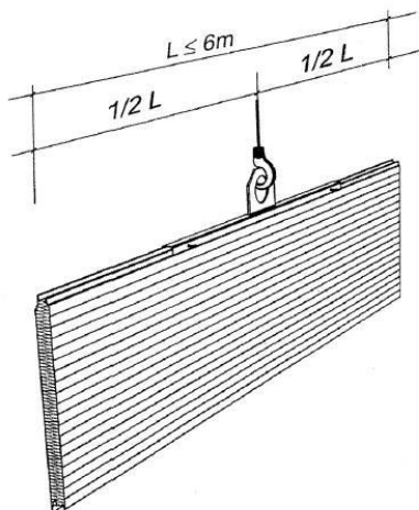
Pav. 24: Daugiasluoksnių statybinių plokščių kelimo kranu schema kai L \leq 6m
