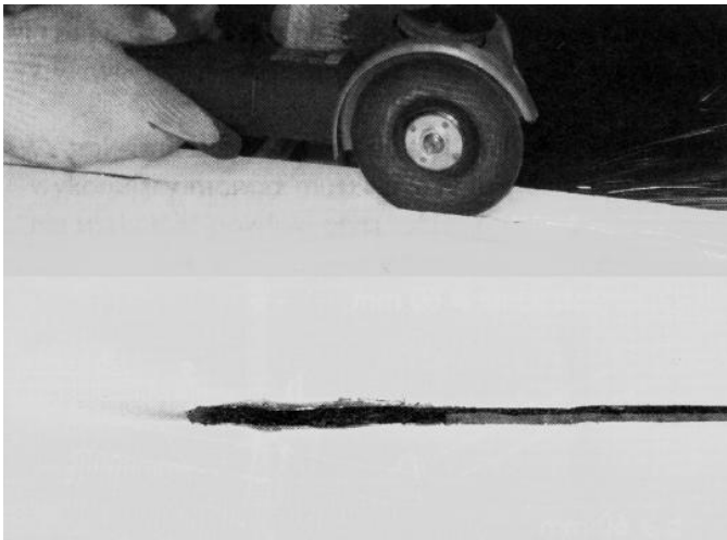
Pav. 7: Daugiasluoksnių statybinių plokščių pjovimui rekomenduojama naudoti metalo pjovimo pjuklus
